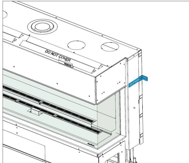
Abb. 10: Befestigung an der Rückwand
