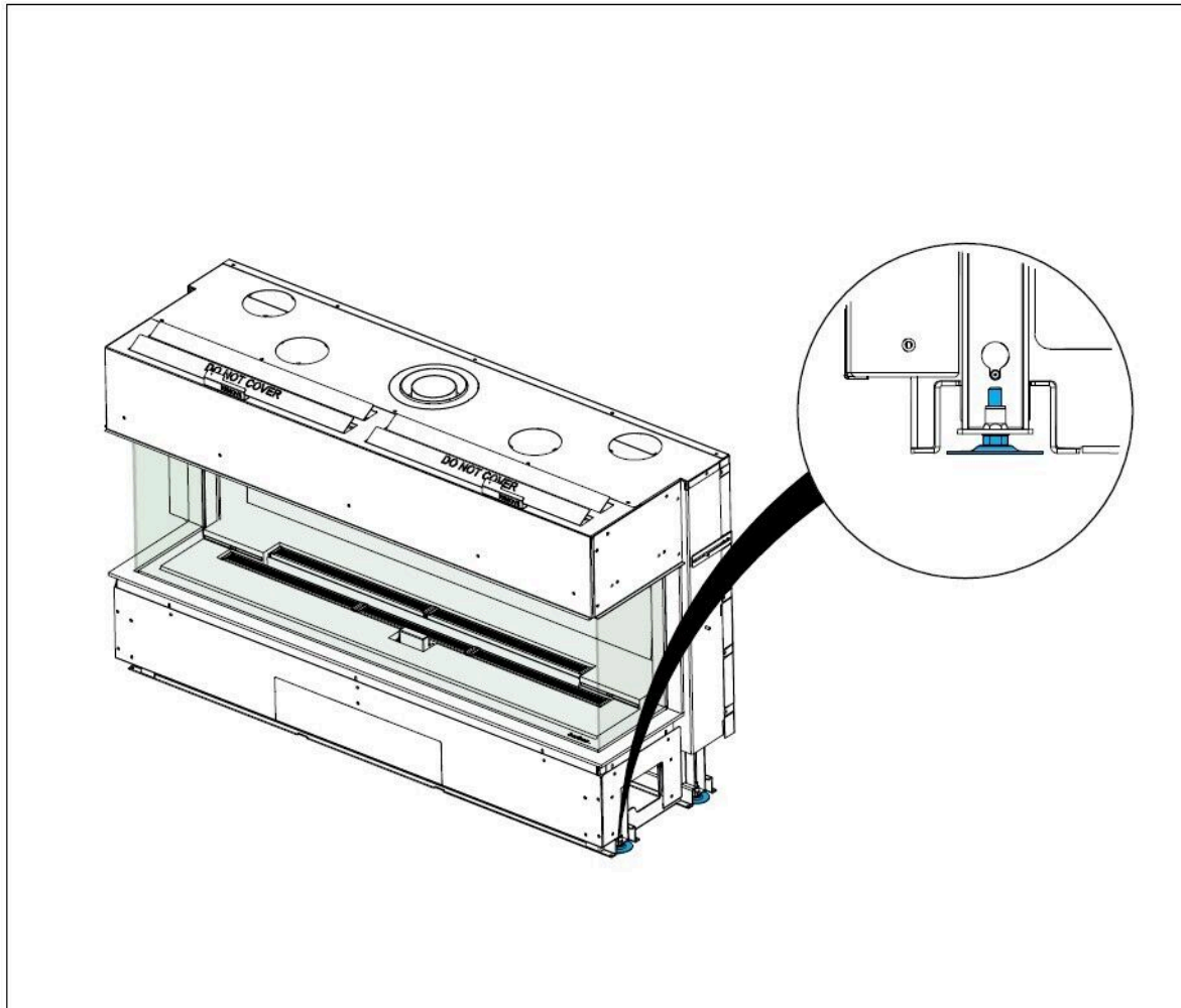
Abb. 8: Ausrichtung mittels Stellfüßen
