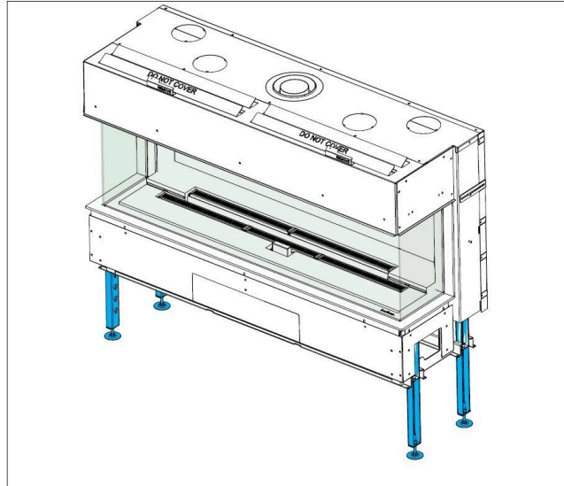
Abb. 9: Ausrichtung mittels höhenverstellbarer Füsse
